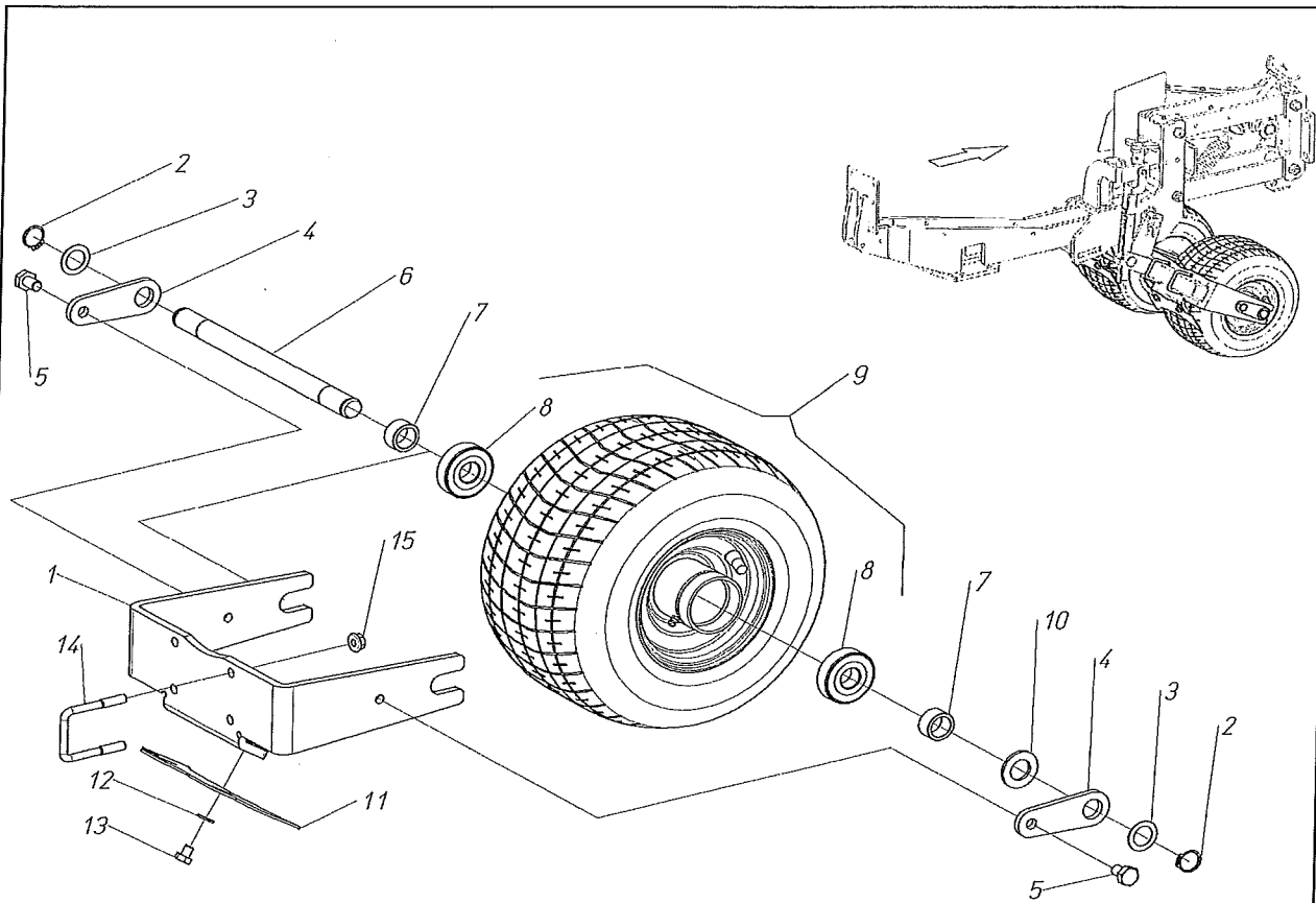
500772 - KIT APPLICAZIONE RUOTA 285x180 SU GOLD
